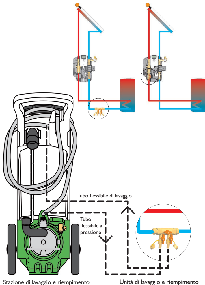
Stazione di lavaggio e riempimento
