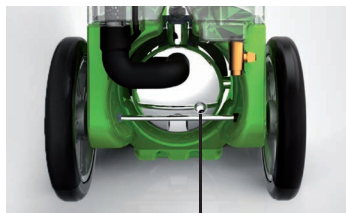
Vite di sfianto
