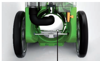
Entlüftungsschraube
